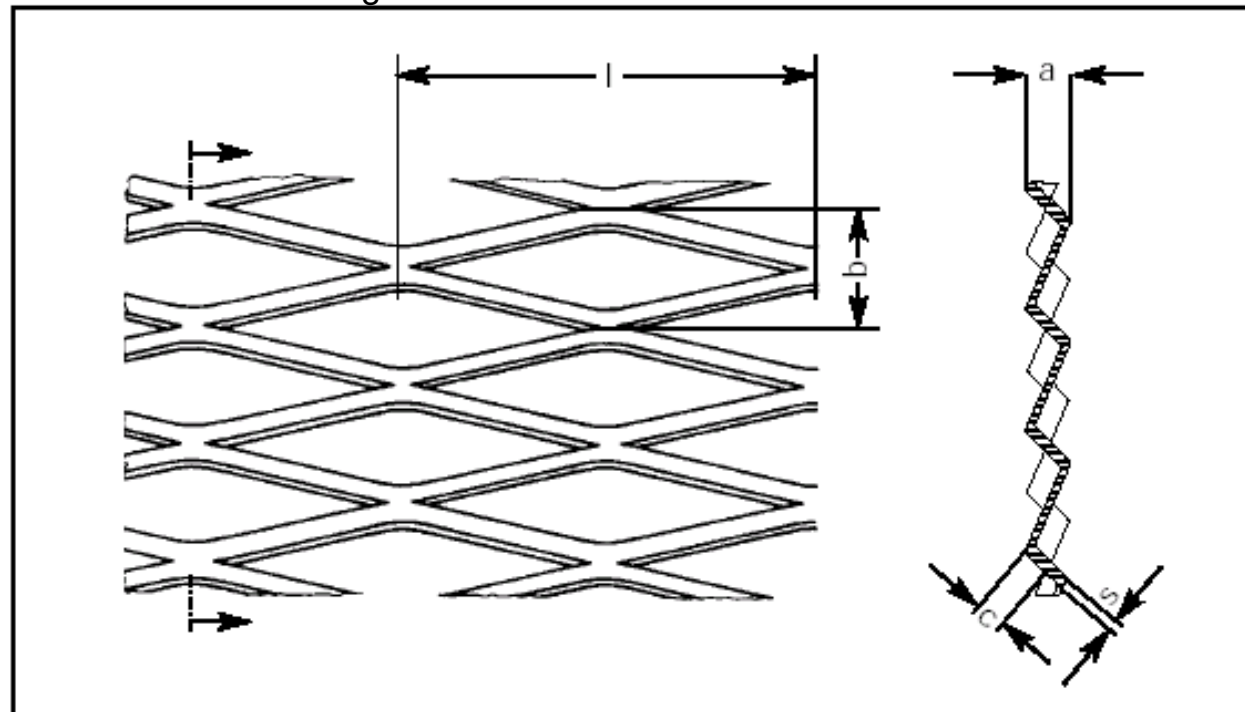
Maschenbeschreibung
